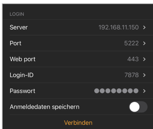
Abbildung 16 – Login-Einstellungen
